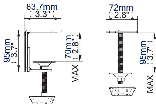
Grommet
