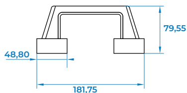
WYMIARY UCHWYTU MAGNETYCZNEGO
