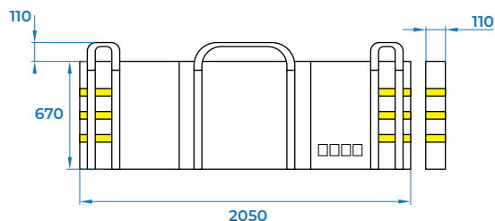
WYMIARY TORBY
